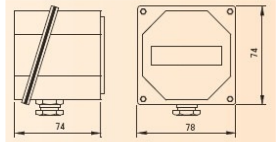
Aansluitkap P3
